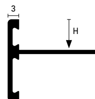
Sezione Alluminio
