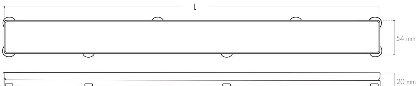
STL-CTF, cover piastrellabile con vaschetta di contenimento
