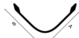
Sezione Alluminio
