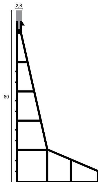
Sezione quotata scala 1:1
