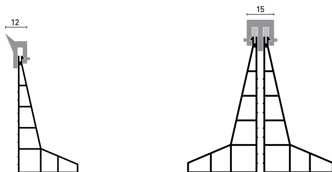
Sezione quotata scala 1:2
