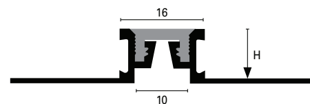
Sezione quotata scala 1:1 (CB 100*)
