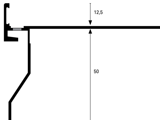
Sezione quotata scala 1:1,2 (BCO 50 A*)
